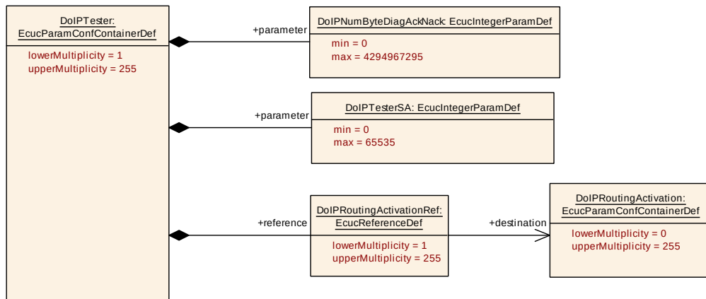
Figure 10.12: DoIPTester
