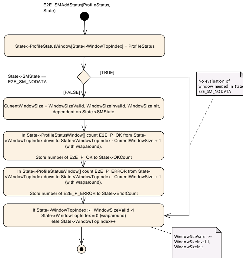
Figure 6.133: E2E state machine step E2E_SMAAddStatus
