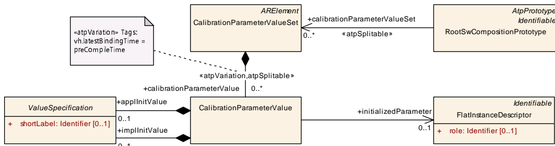
Figure 5.69: Calibration Parameter Values
