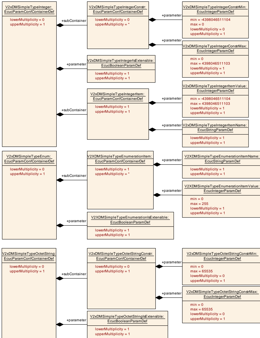
Figure 10.14: V2xDMMMessageSimpleTypes2
