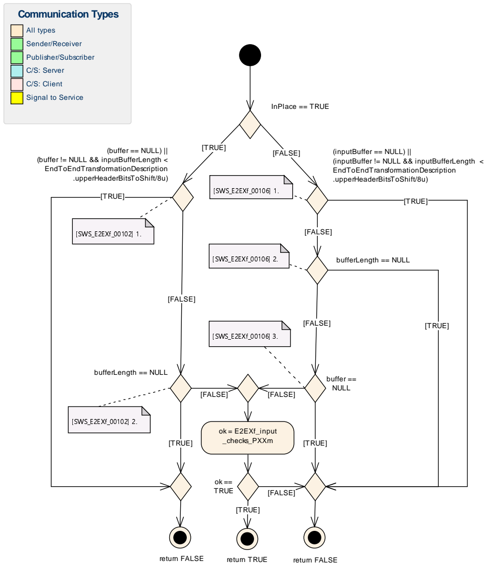
Figure 7.3: E2EXf_input_checks()
