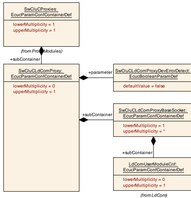
Figure 10.34: LdCom Proxy Parameter
