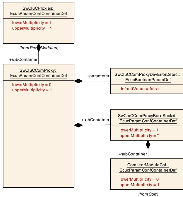
Figure 10.29: Com Proxy Parameter
