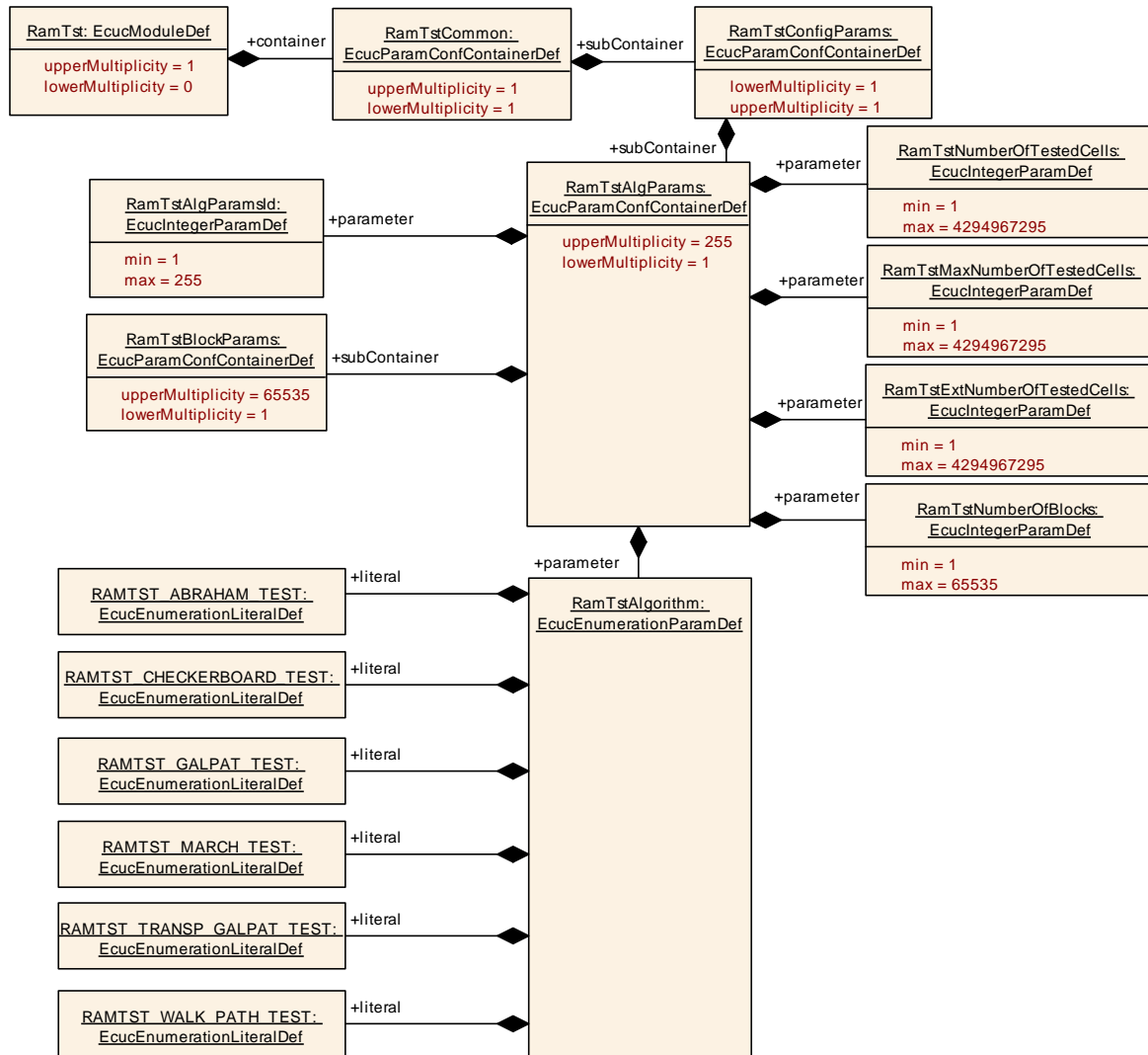
Figure 18: RamTstAlgParams
